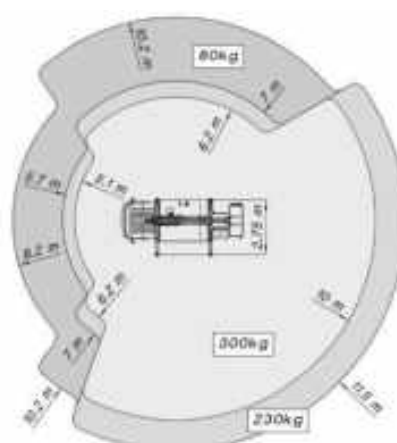
Abstützung einseitig
