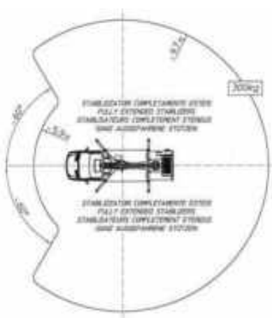
Abstützung beidseitig
